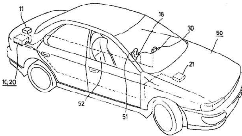
車両に取付けた例を示す図
