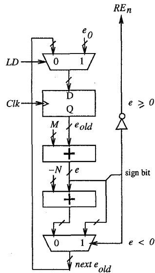
Figure 10: The E Gen module.
