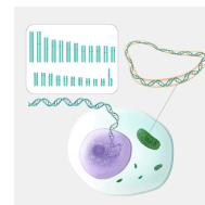
Genome
