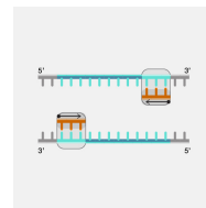
Primer
