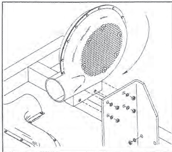
BLOWER ROTATION
