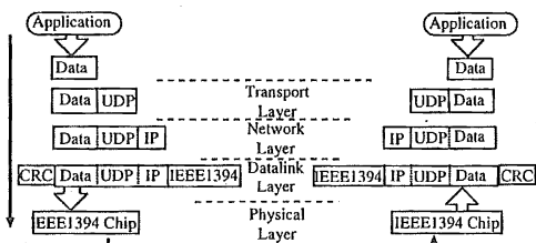
Fig. 4 UDP/IP protocol suite.
