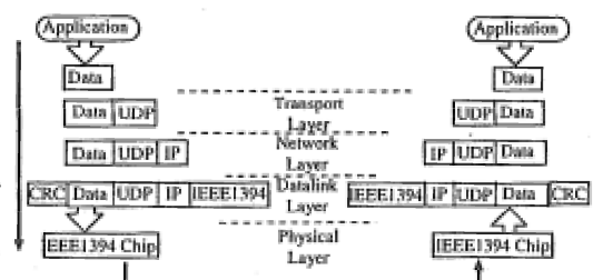
Fig. 4 UDP/IP protocol suite.
