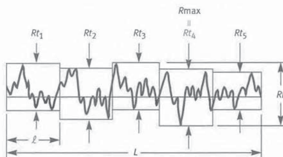
Fig. 1-11 The R_t and R_{\max} Parameters
