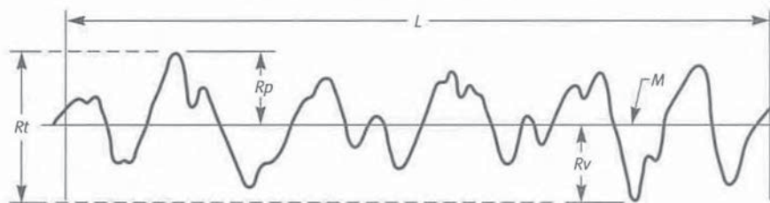
Fig. 1-9 R_t , R_p , and R_v Parameters
