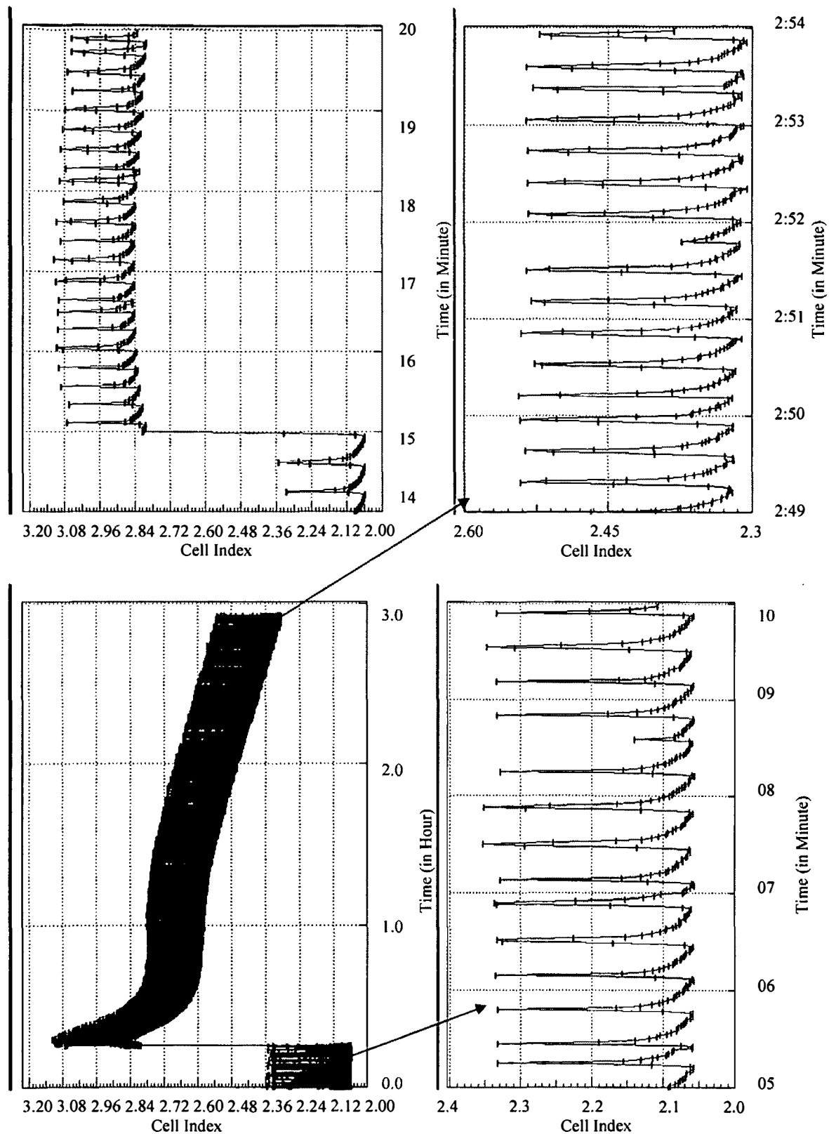
FIG. 11S DMSO 0.13%
