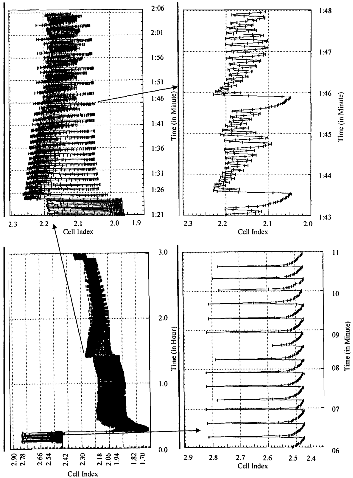
FIG. 110 E4031 9.1 nM
