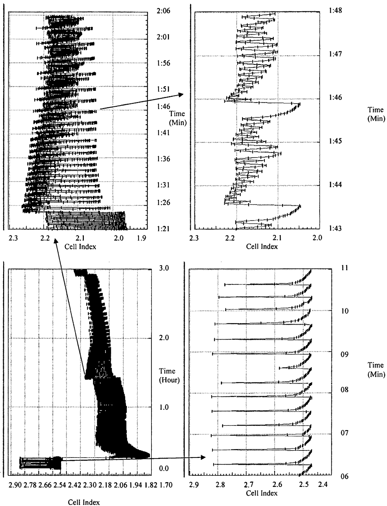
FIG. 110 E4031 9.1 nM
