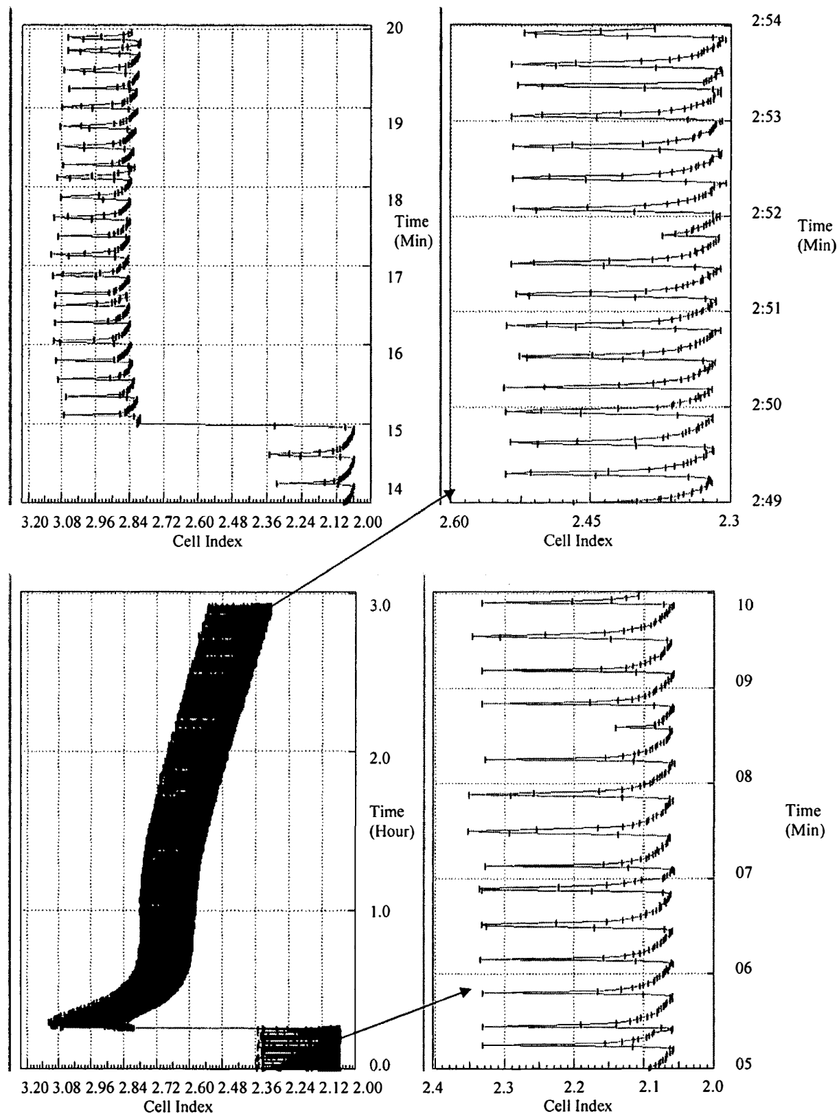
FIG. 11S DMSO 0.13%
