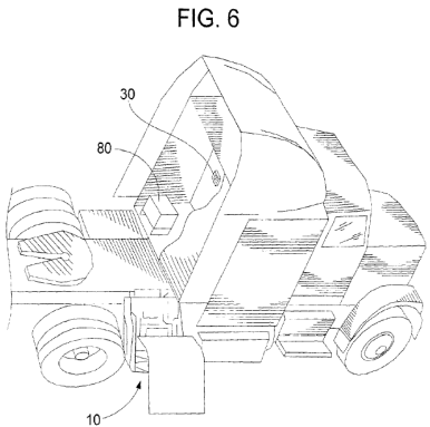
Ex. 1009 (Zeigler), Fig. 6 (non-electric)
