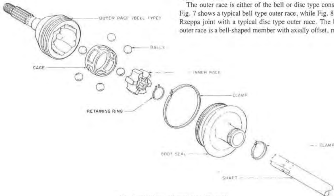
Fig. 7 — Rzeppa universal joint (bell type)
