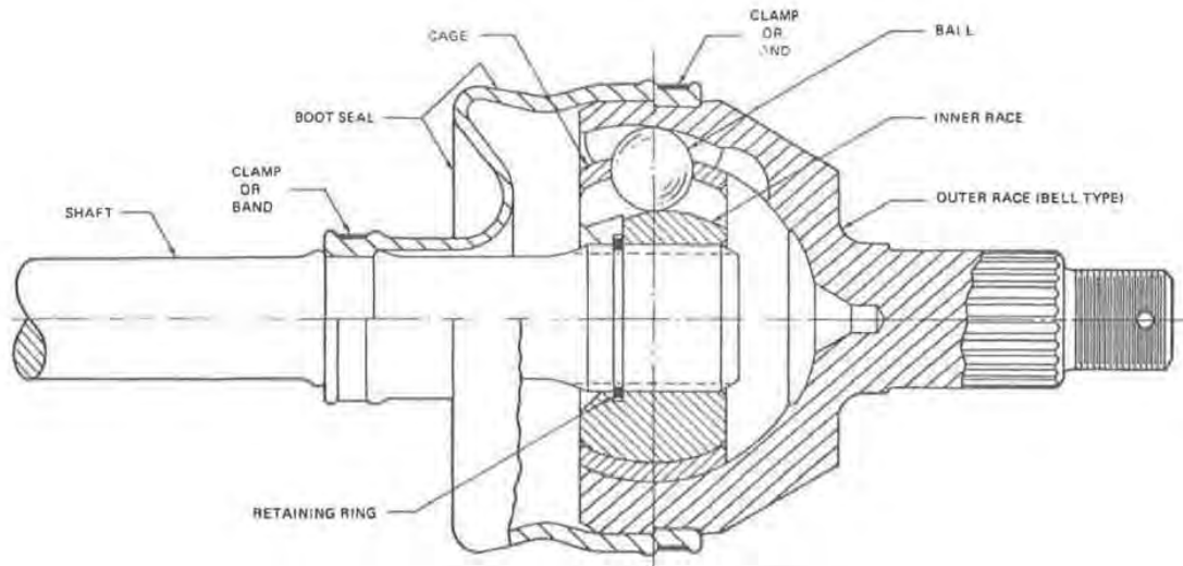
Fig. 1 — Rzeppa universal joint (bell type)
