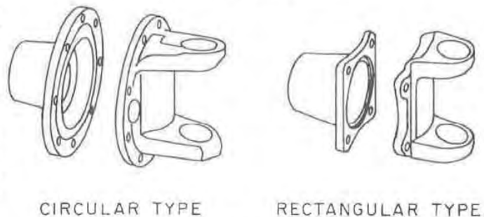
Fig. 6 — Flange yoke
