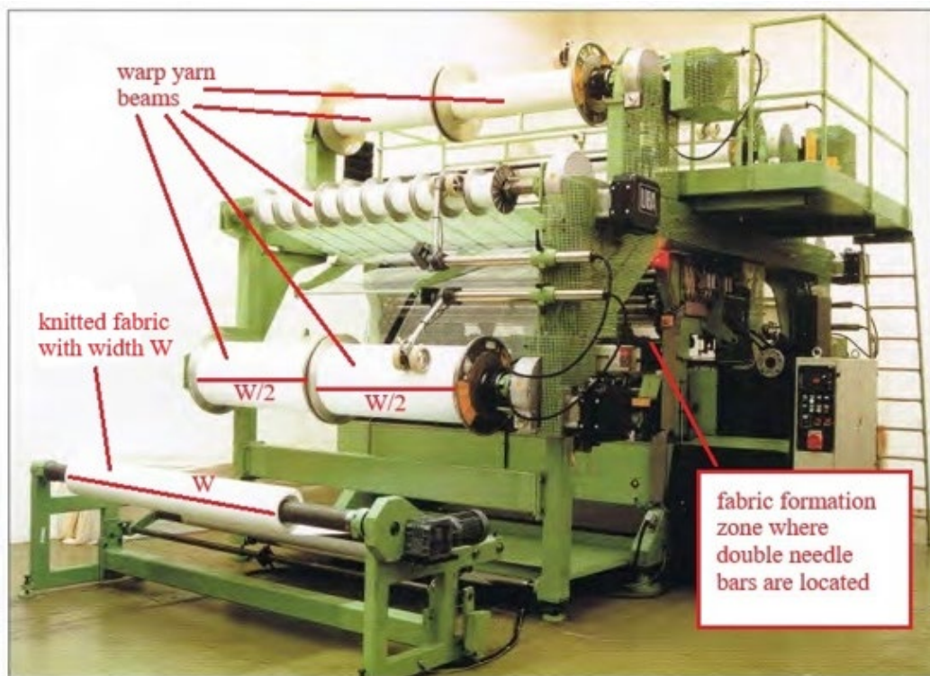
Doppelnadelbarrige Raschelmachines Double Needle Bar Raschel Machines
