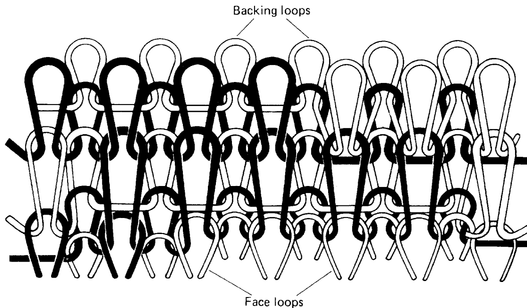
Fig. 10.6 Rib jacquard.
