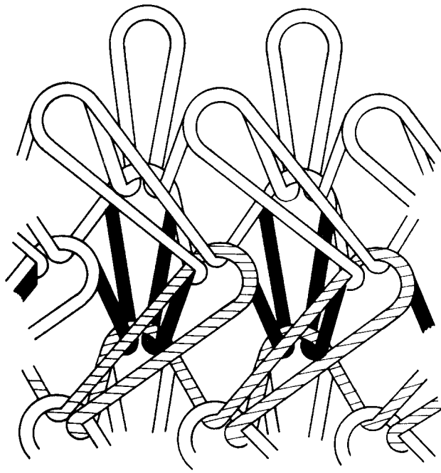
Fig. 18.7 Raked rib.
