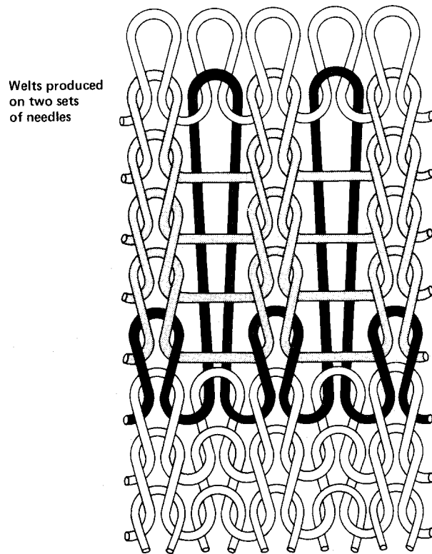
Fig. 16.5 Roll welt.
