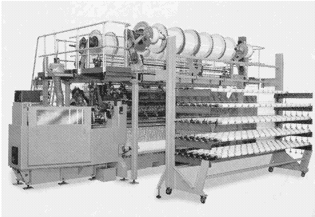
Fig. 28.17 Textronic MRPJ 59/1/24 raschel lace machine [Karl Mayer].
