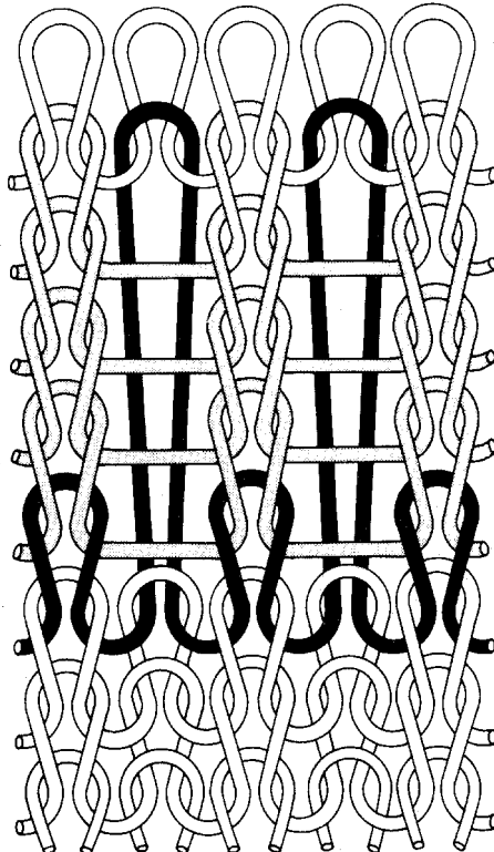
Fig. 16.5 Roll welt.
