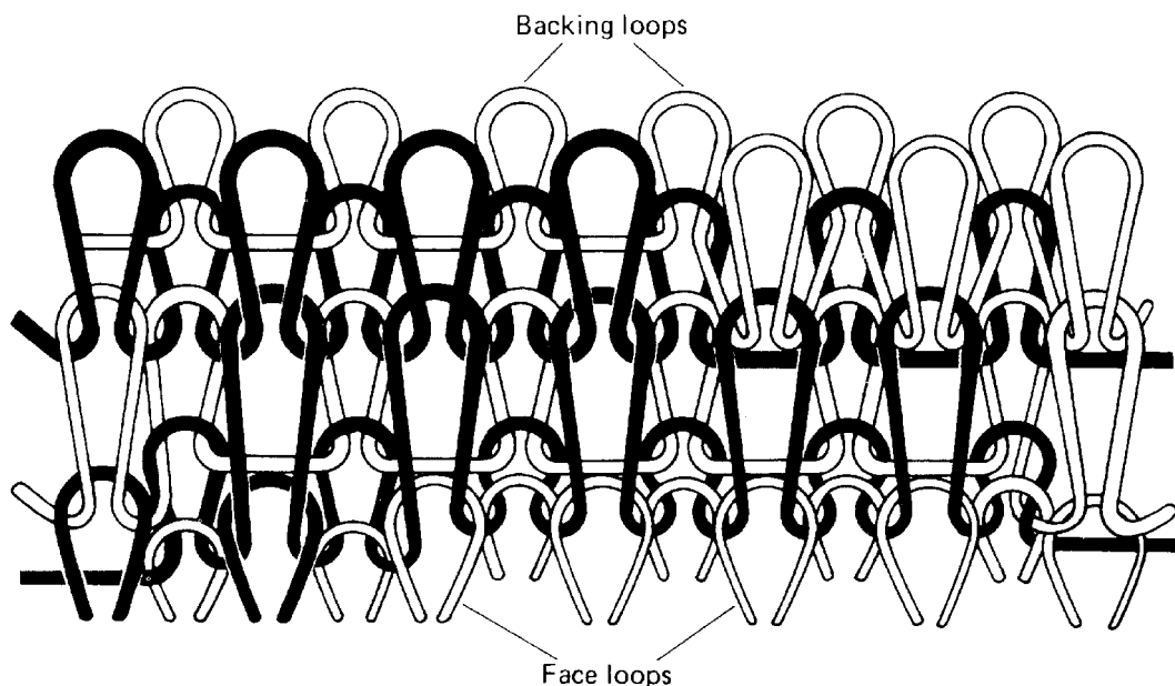
Fig. 10.6 Rib jacquard.
