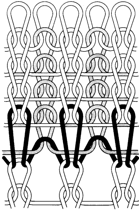
Fig. 16.4 Tubular welt.
