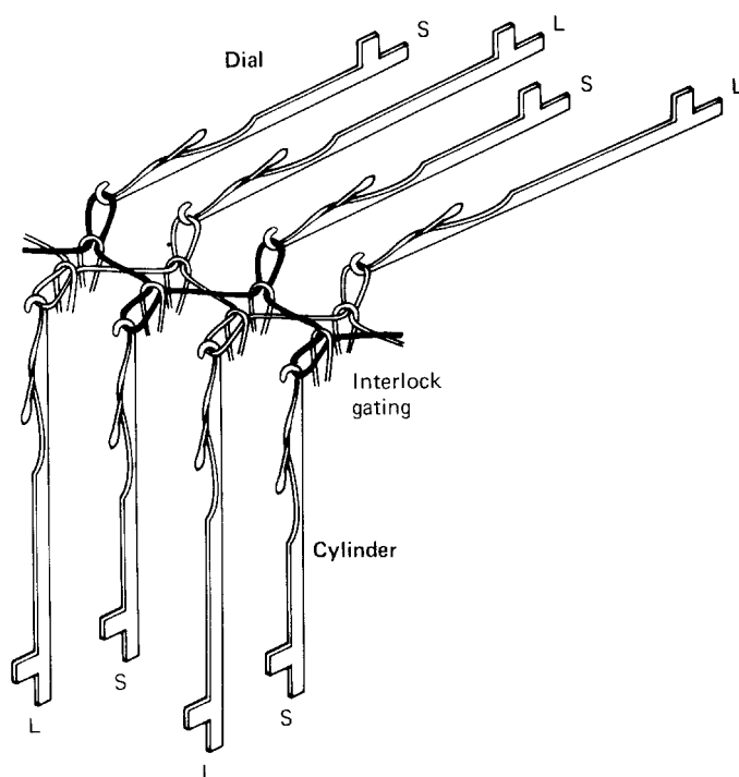
Fig. 7.15 Knitting interlock.
