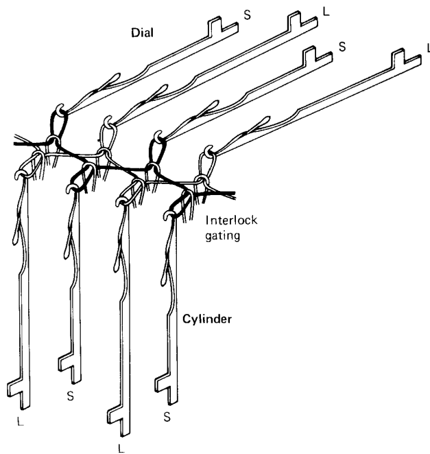
Fig. 7.15 Knitting interlock.
