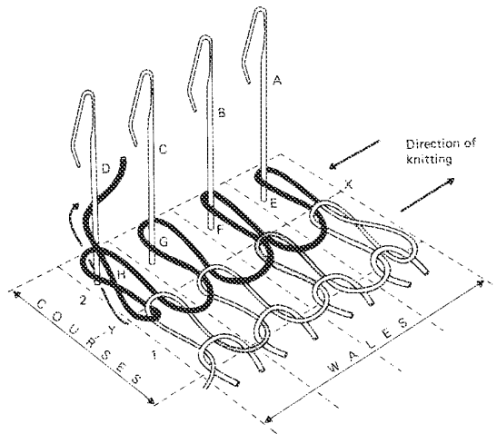
Fig. 6.1. Weft knitting
