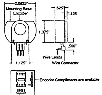
Optical Encoder (EN)
