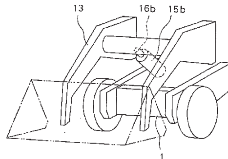
リフトシリンダの第3取付例を示す斜視図
