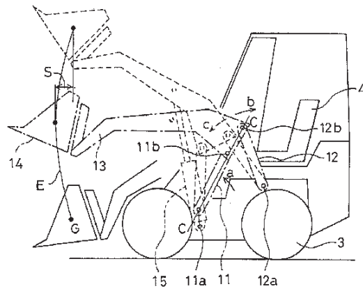
第1実施例の作動説明図
