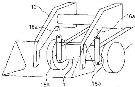
リフトシリンダの第2取付例を示す斜視図
