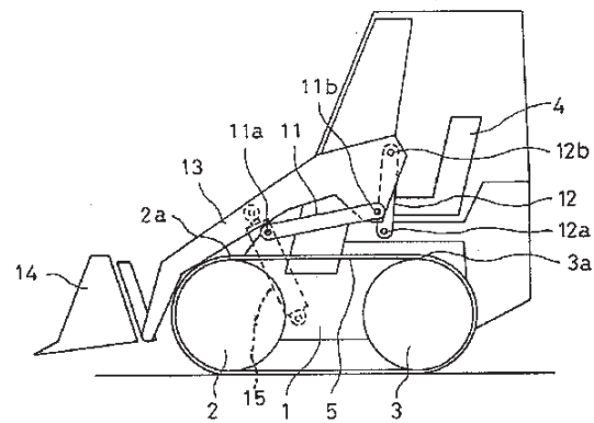
第2実施例の4節リンクを備える作業車両の側面図
