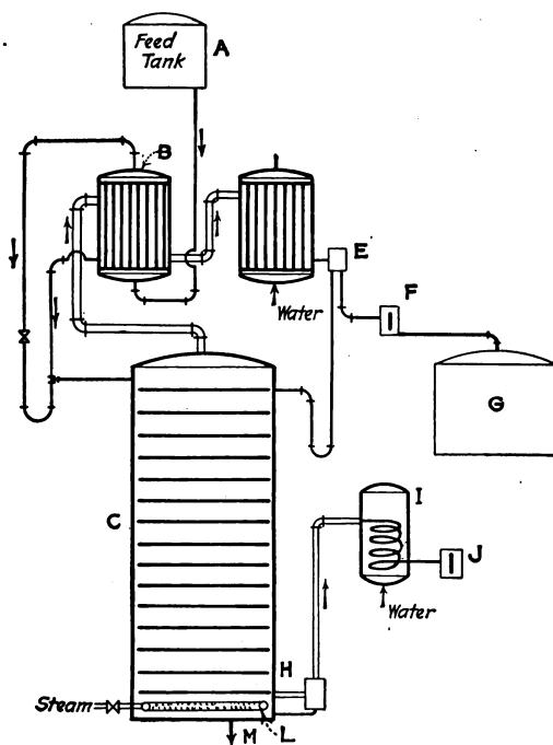
FIG. 37.—Beer still.
