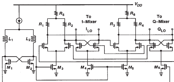
Fig. 3. LO/divider circuit.
