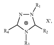
Triazolium
