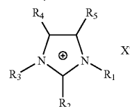
Imidazolium
