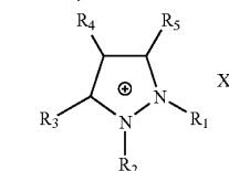
Pyrazolium
