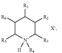
Piperidium
