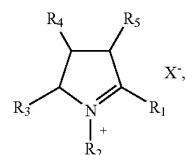
Pyrrolinium
