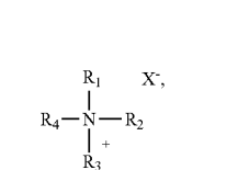
Ammonium
