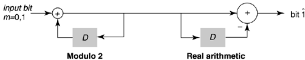
Figure 2.6. Encoder/ modulator for AMI.
