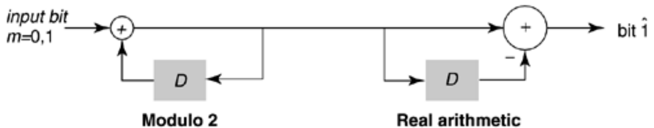
Figure 2.6. Encoder/ modulator for AMI.
