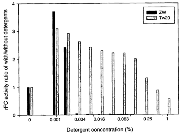
FIG. 1. Zwittergent 3-14 and Tween 20
