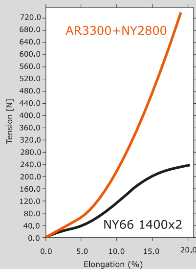
Tensile Strength
