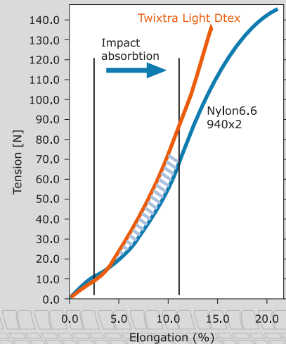
Tensile Strength
