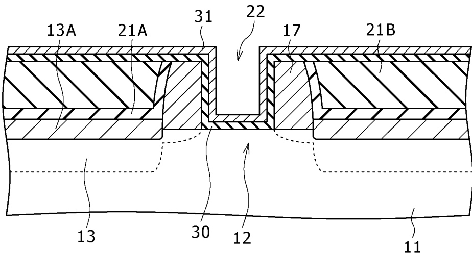
FIG. 2E [PROCESS-210]
