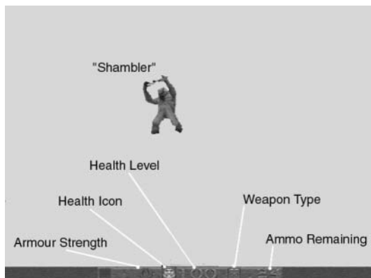
Fig. 8. Status bar.
