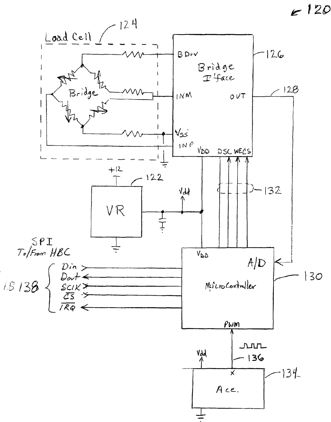
FIG. 4 Pedal Sensor Module
