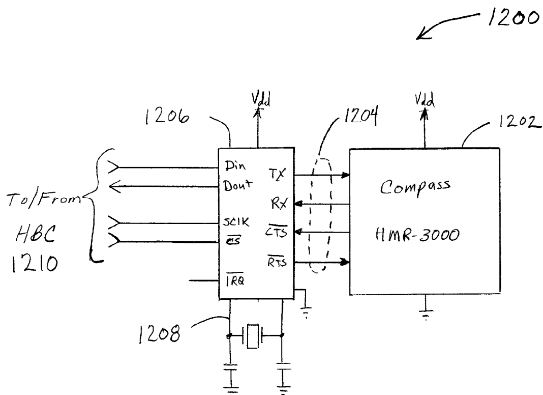
FIG. 23 Compass Module
