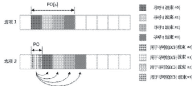
• 图 2.基于多波束操作的寻呼示例
