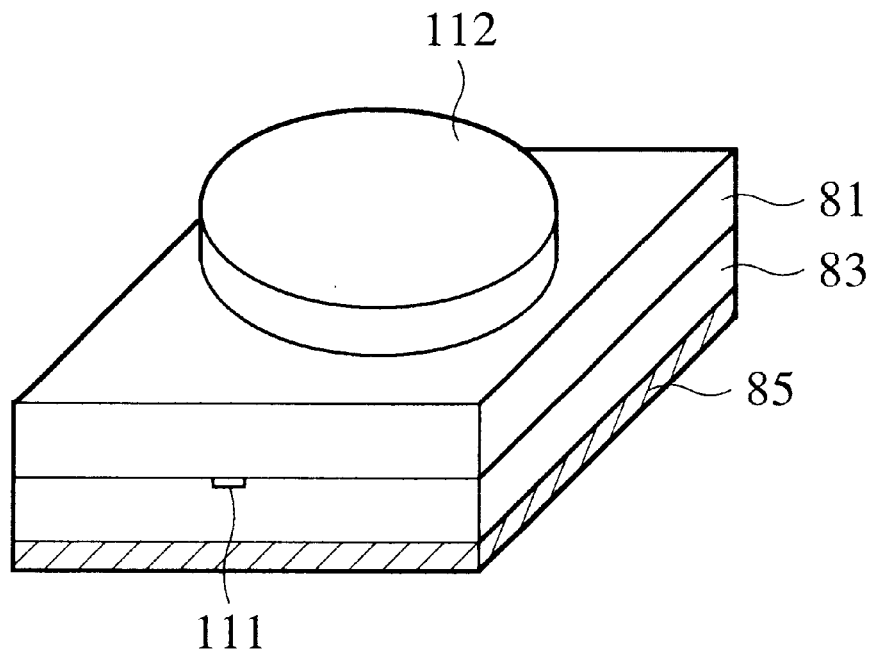
FIG.37A
