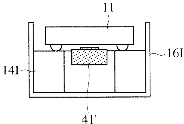
FIG.20B
