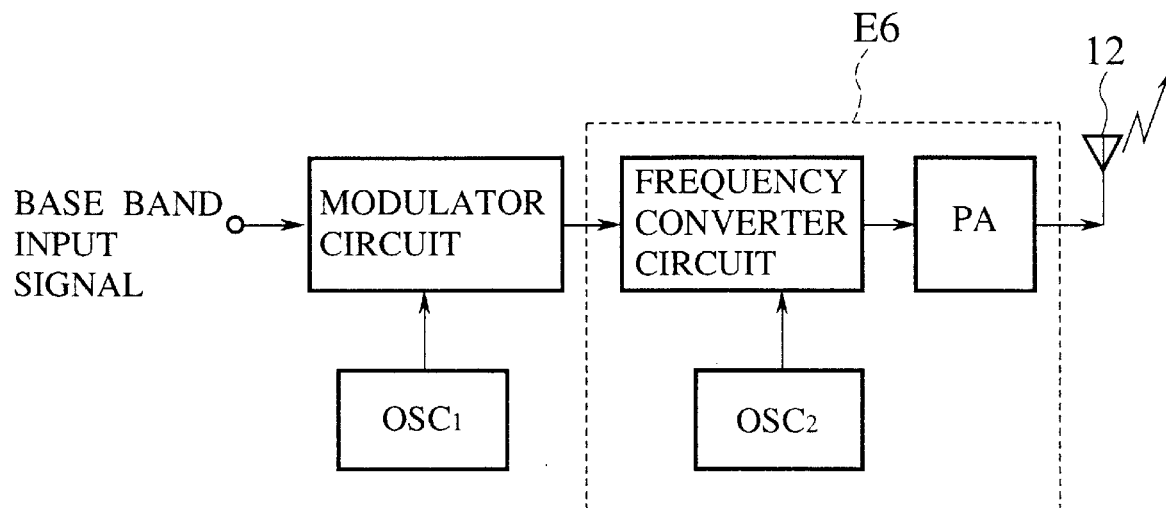
FIG.31
