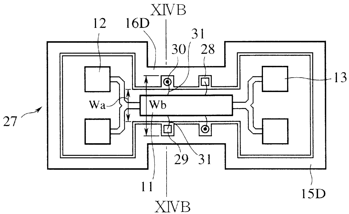
FIG. 14A
