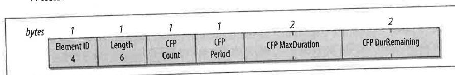
Figure 8-9. CF Parameter Set information element
