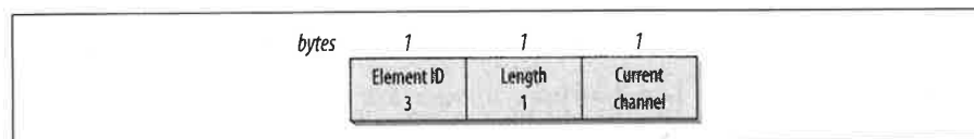
Figure 4-35. DS Parameter Set information element
