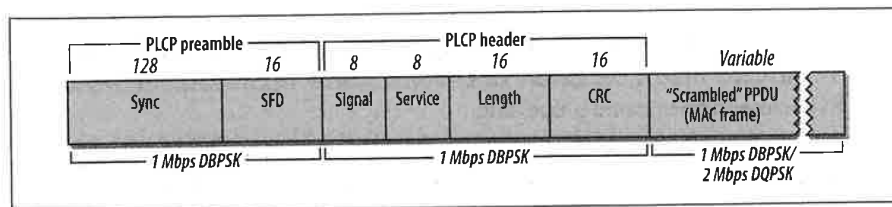
Figure 10-23. DS PLCP framing
