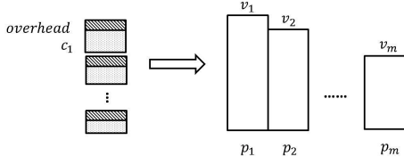
Fig. 3. Virtual Knapsack
