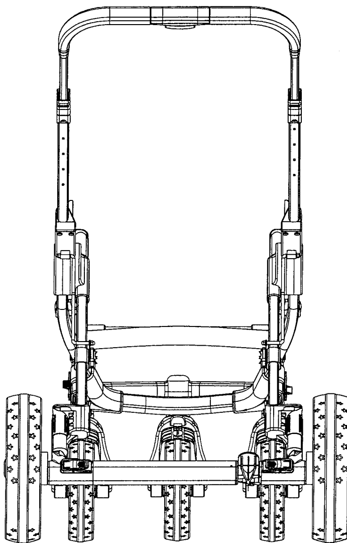
後視圖
