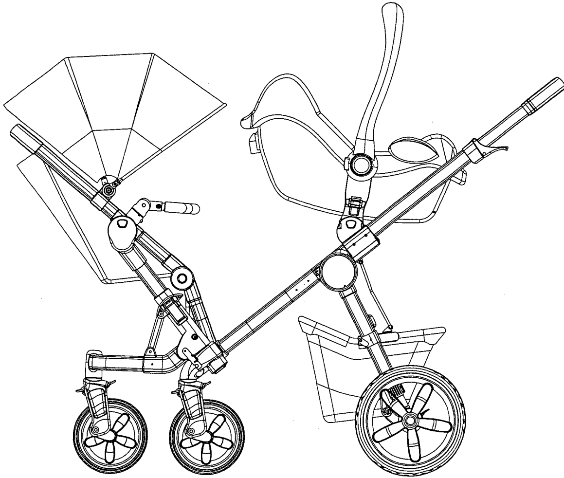
本創作加裝置物籃+安全座椅+座艙 之使用狀態參考圖
