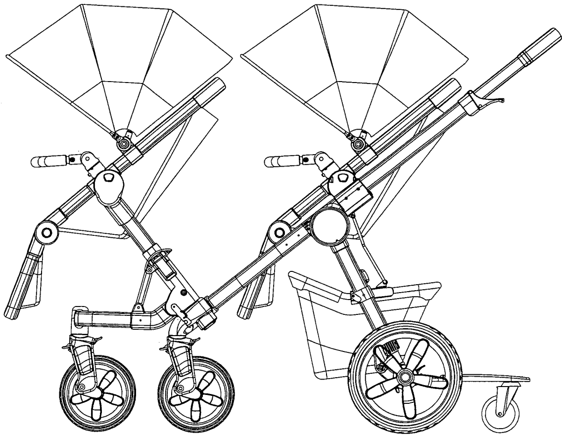
本創作加裝置物籃+兩座艙+滑板 之使用狀態參考圖(一)
