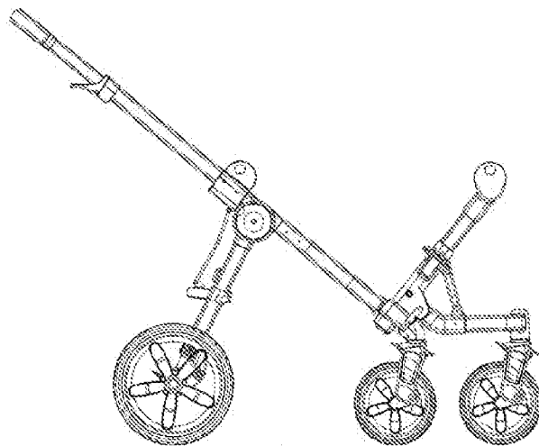
左側視圖
