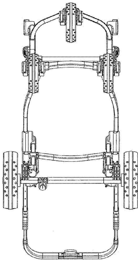
仰視圖
