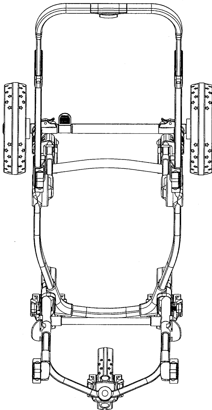
俯視圖
