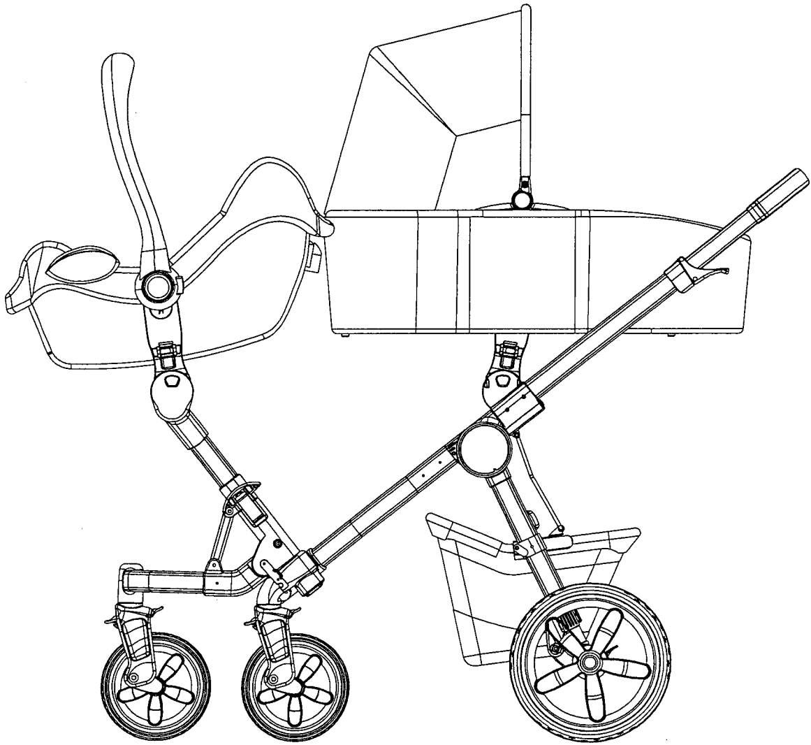
本創作加裝置物籃+安全座椅+手提睡籃 之使用狀態參考圖
