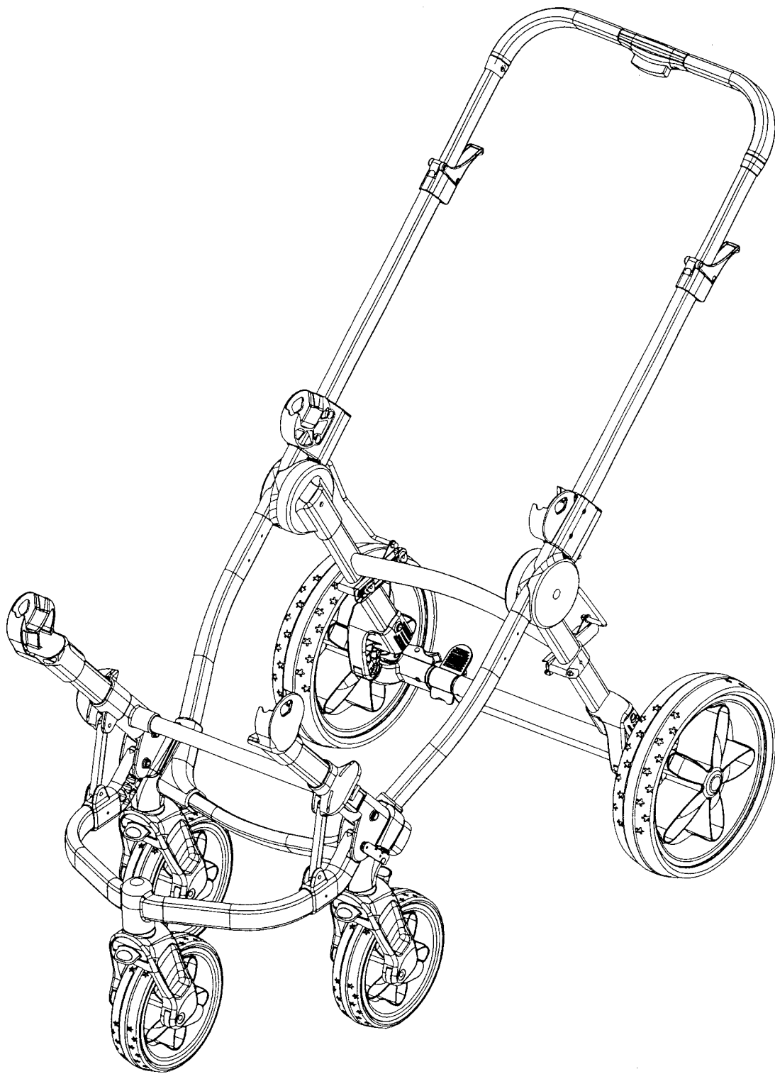
立體圖(代表圖)
