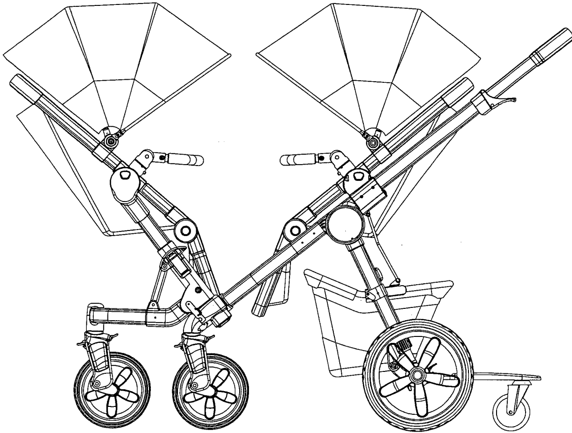
本創作加裝置物籃+兩座艙+滑板 之使用狀態參考圖(二)
