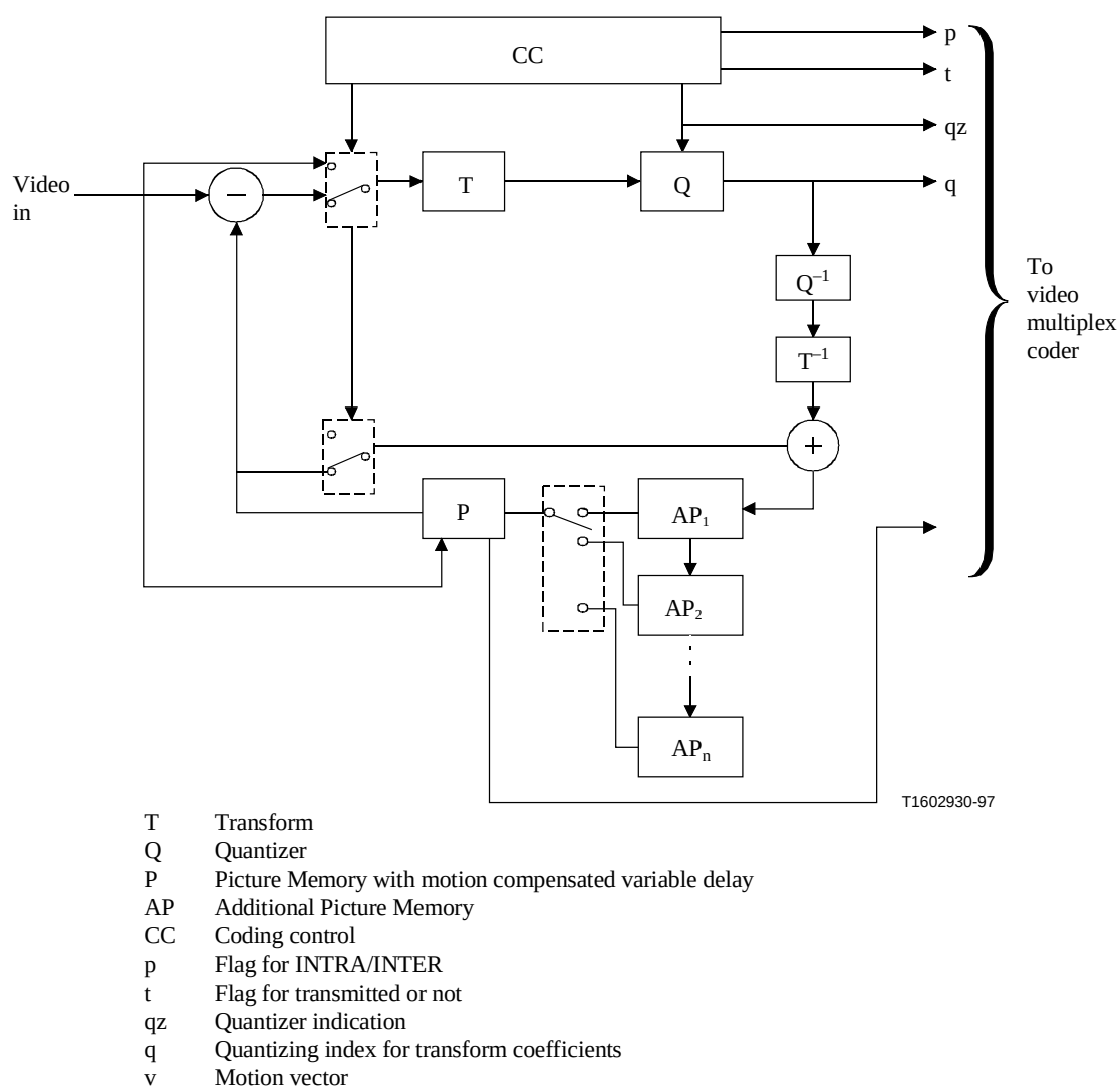
Figure N.1/H.263 – Source coder for NEWPRED
