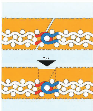
Fig. 11. Ett glapp på några 1/10-dels millimeter i den snett uppskurna vadden betyder minskad materialmängd längs flera millimeter i maskinriktningen. Detta kan innebära risk för markering i pressrytet.
