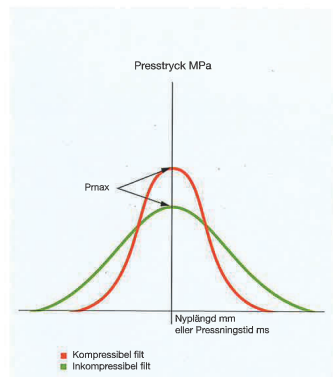
Fig. 1. Klockkurvor f6r tryckets f6rdelning genom pressnypet.
