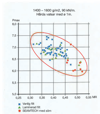
Fig. 2. Maxtrycket i mittnypet som funktion av fuktkvoten, MR, av m6ttad filt komprimerad till maxtrycket. En skara filter visas vid samma linjetryck och i samma nyp fr6n kompressibla med MR = 0,3 till inkompressibla med MR = 0,5.
