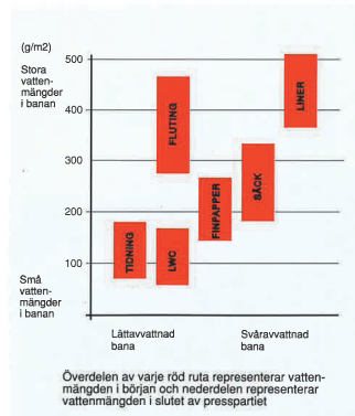
Fig. 3. N6gra papperssorter ordnade i ett samband d6r pressningen blir mer tryckberoende ned6t mot v6nster och mer fl6desberoende upp6t mot h6ger. N6gon skarp gr6ns finns inte.
