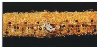
Fig. 10. Avancerad söm med fiberförankring också på öglorna enligt patentsökt förfarande.
