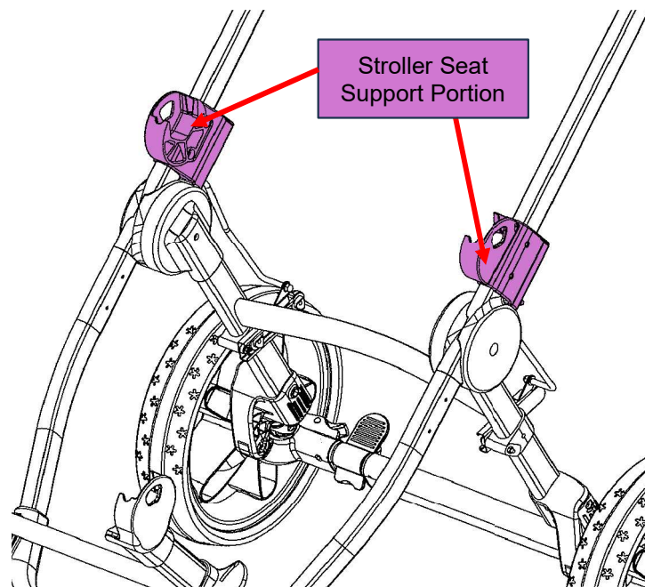
EX1051, Liao, Fig. 1
