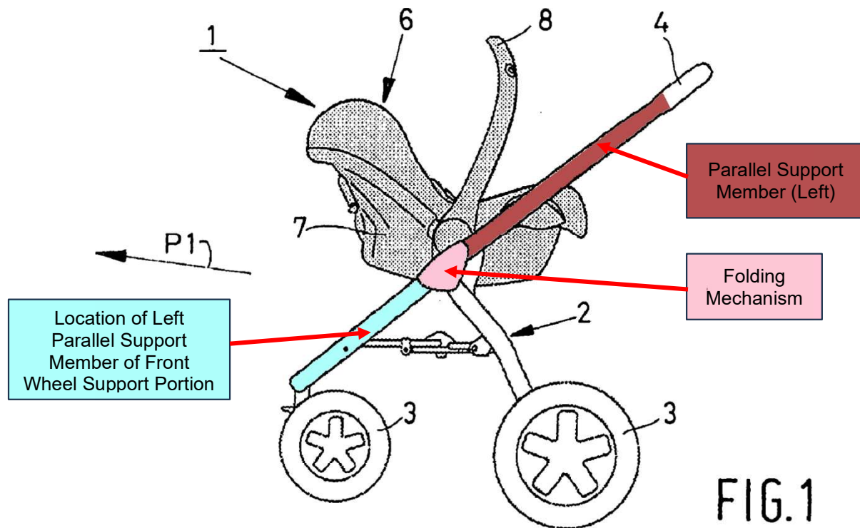
EX1050, Van Dijk, Fig. 1
