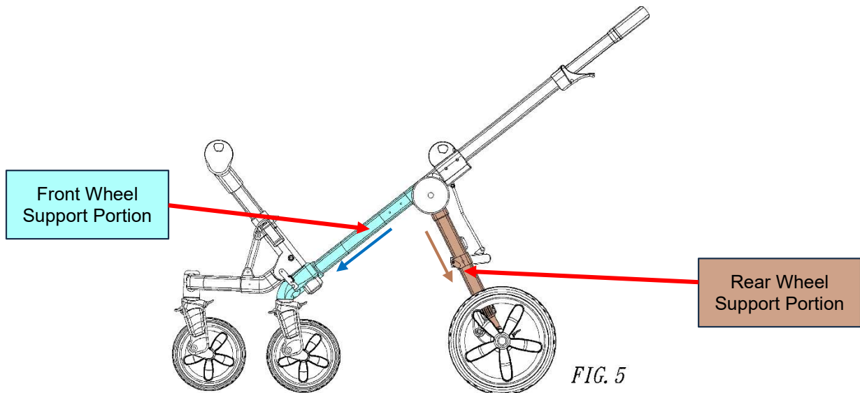
EX1051, Liao, Fig. 5
