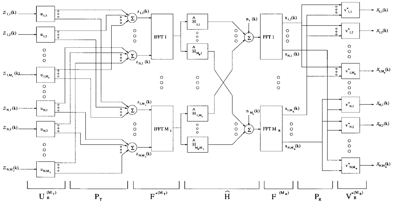
Fig. 4. DMMT system diagram.
