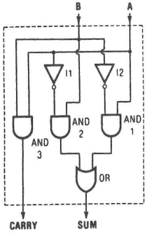
Circuit.
