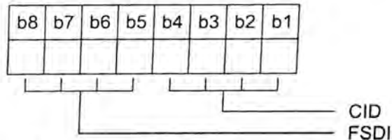
Figure 3 — Coding of RATS parameter byte
