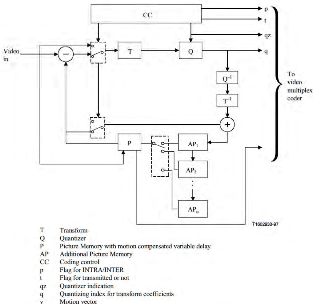
Figure N.1/H.263 – Source coder for NEWPRED
