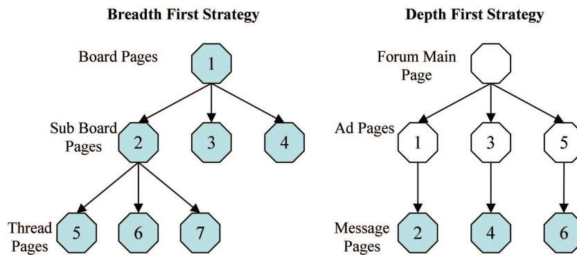
FIG. 3. URL traversal strategies.
