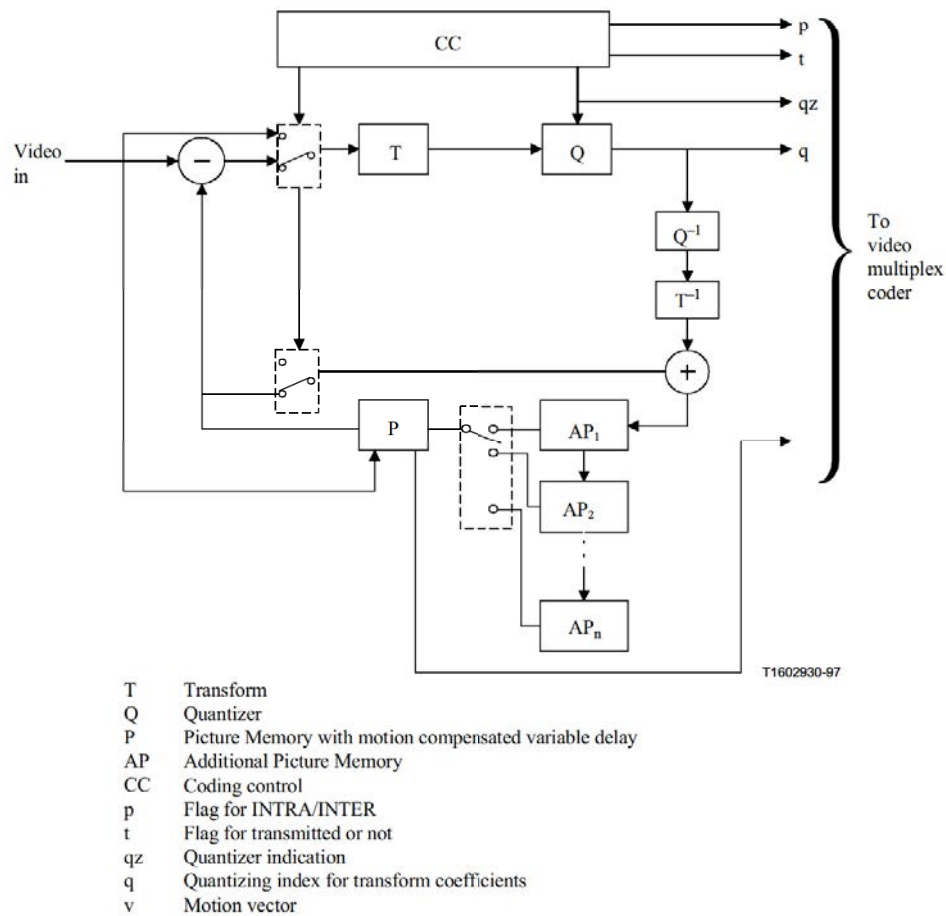
Figure N.1/H.263 – Source coder for NEWPRED
