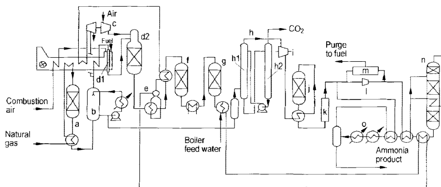
Figure 110. ICI AMV process
