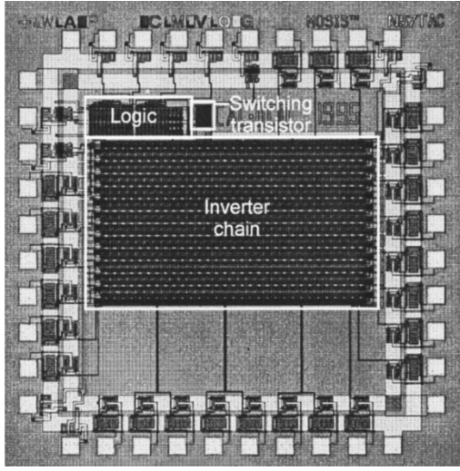
Fig. 6. Test chip die photo.
