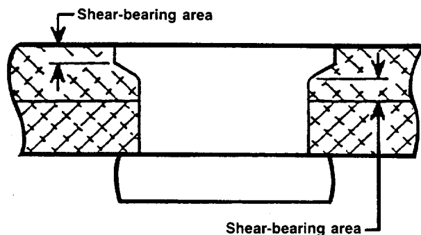
Figure 35.—BRZF 'fast' rivet.
