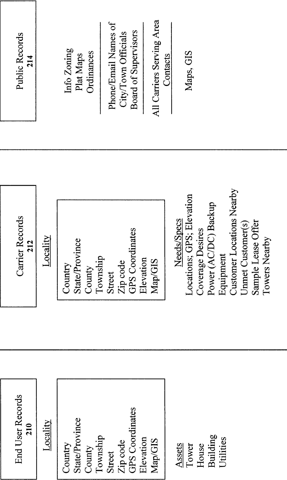
Fig. 2 All Records
