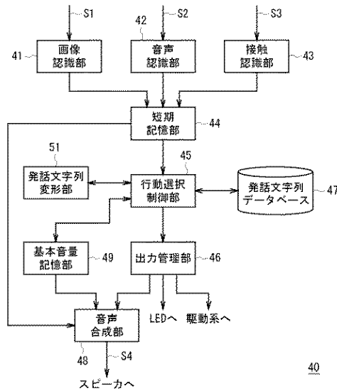
図 4 本実施の形態によるロボットにおける行動制御システムの構成
