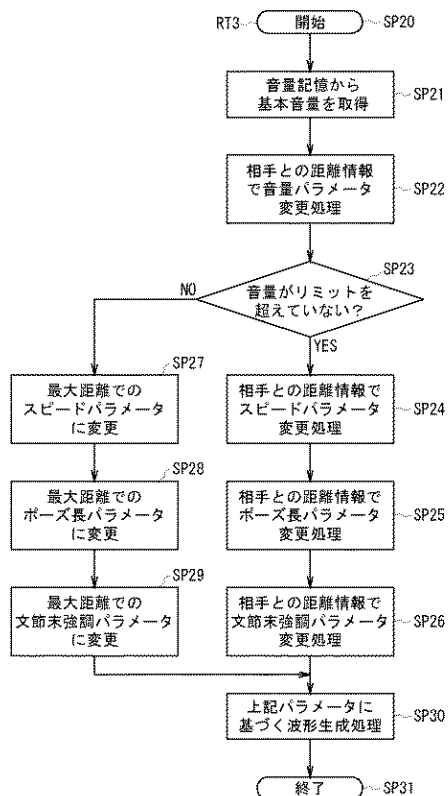
図 13 発話変更処理手順
