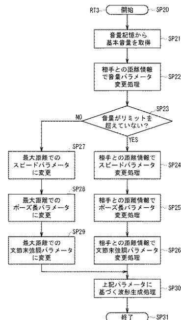
図13 発話変更処理手順
