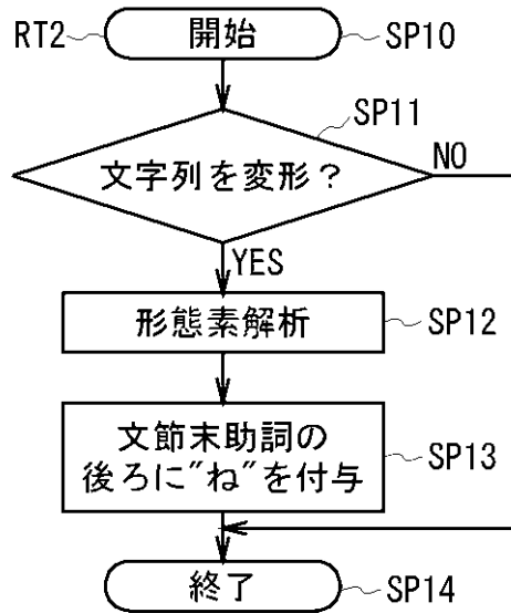
図 8 文字列変形処理手順
