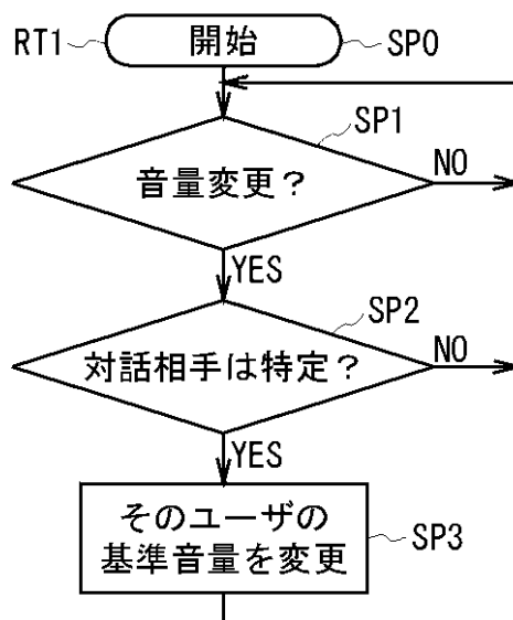
図 6 基準音量変更処理手順
