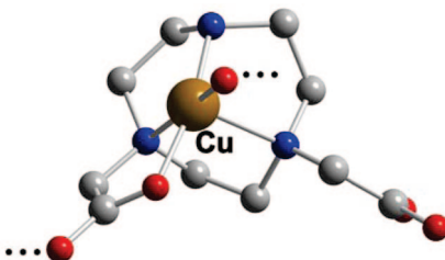
Figure 12. Cu-NO2A (L28).
