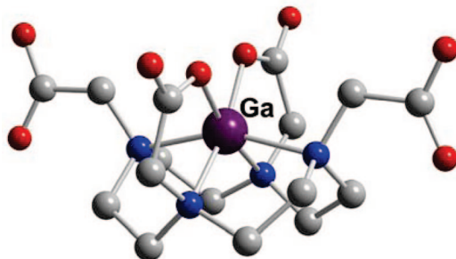
Figure 38. Ga-DOTA (L39).
