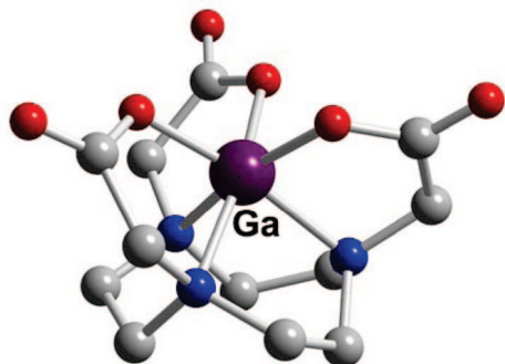
Figure 36. Ga-NOTA (L29).
