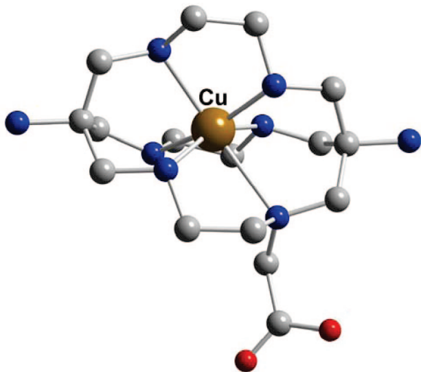
Figure 28. Cu-L63.
