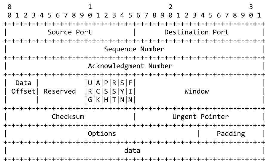
TCP Header Format
