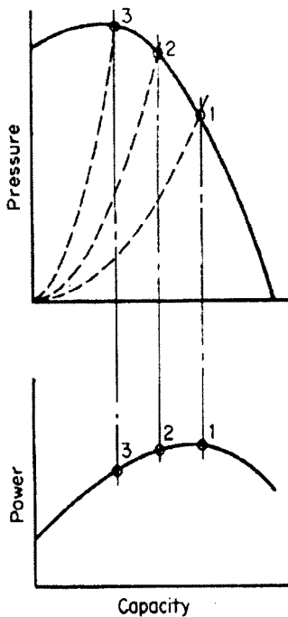
Fig 12-22. Non vortex damper
