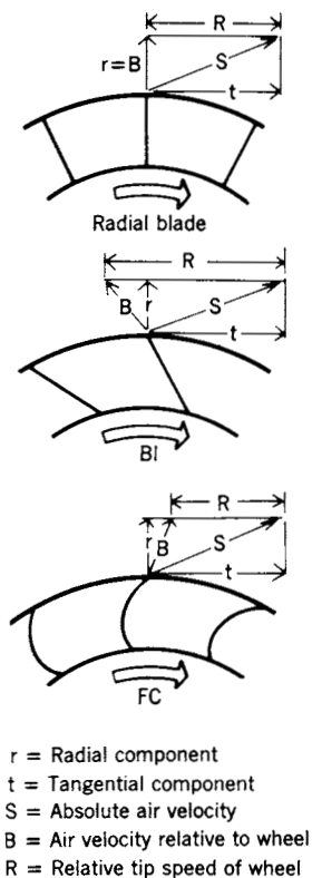
Fig 14-32. Centrifugal fan wheels
