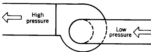
Fig 14-26. Fan surge
