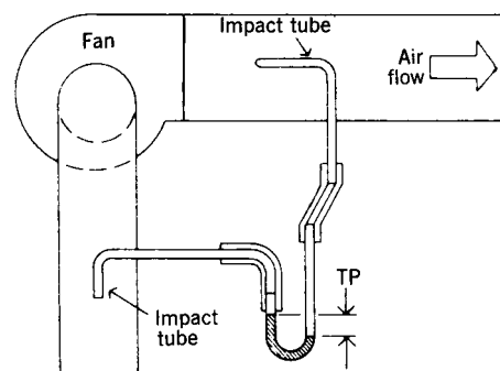
Fig 14-2. Fan total pressure
