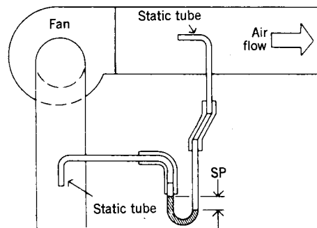
Fig 14-3. Fan static pressure
