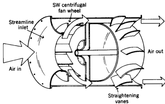
Fig 14-37. Tubular centrifugal fan
