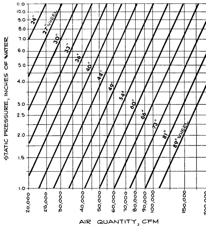
Fig 13-76. Double width fan selection
