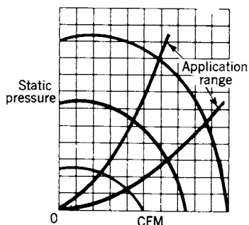
Fig 14-5. Fan curve
