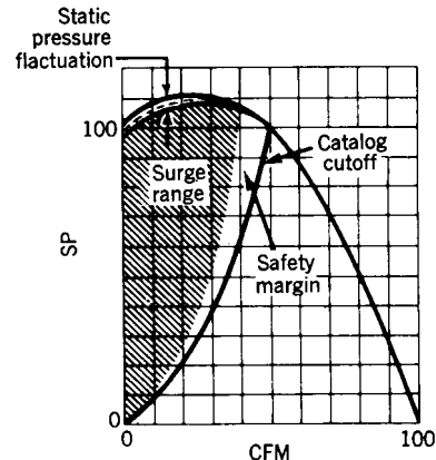
Fig 14-27. Fan surge
