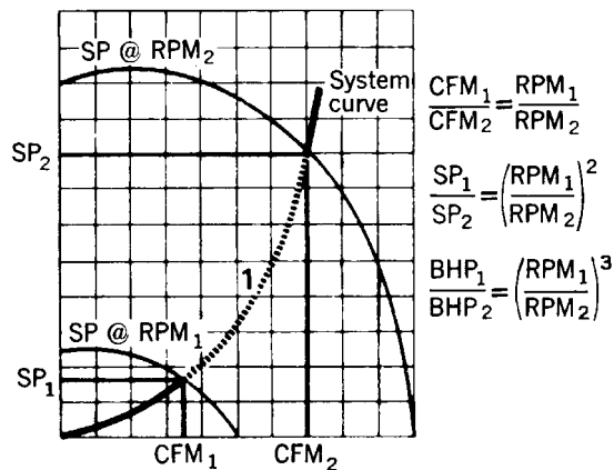
Fig 14-9. Fan law no. 1—RPM change
