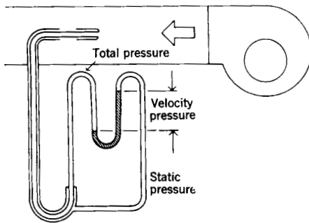
Fig 14-4. Fan velocity pressure
