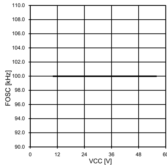
Fig.2 FOSC-VCC
