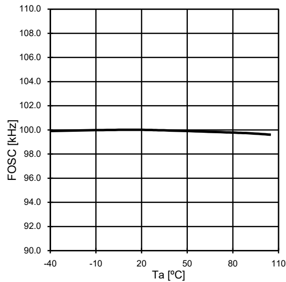
Fig.1 FOSC-Ta
