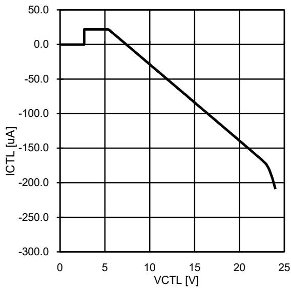
Fig.31 ICTL-VCTL
