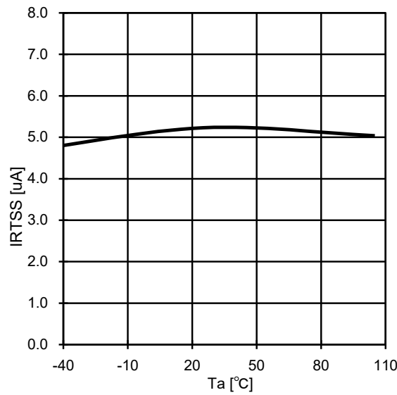
Fig.3 IRTSS-Ta (VRTSS=0V)
