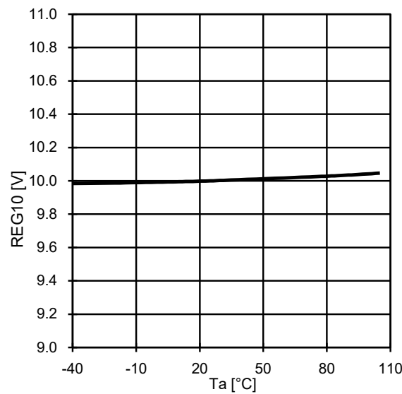
Fig.23 REG10-Ta
