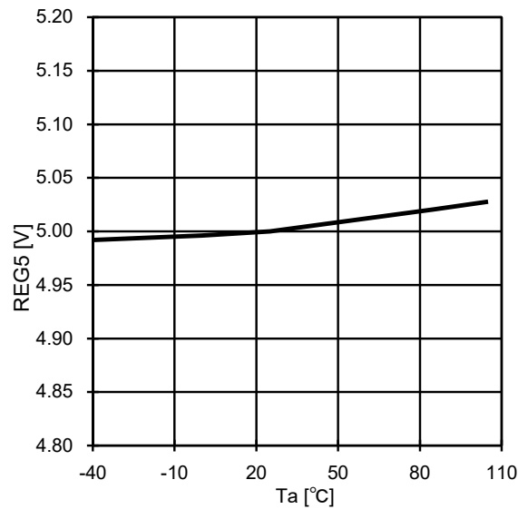
Fig.25 REG5-Ta
