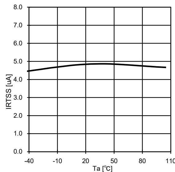
Fig.4 IRTSS-Ta (VRTSS=1V)
