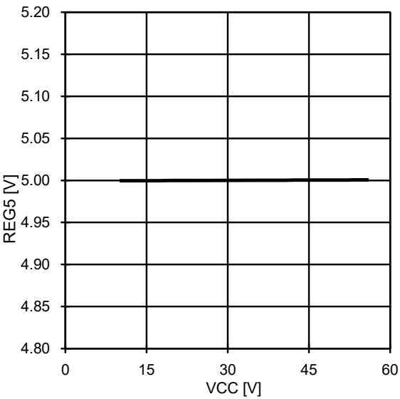
Fig.26 REG5-VCC
