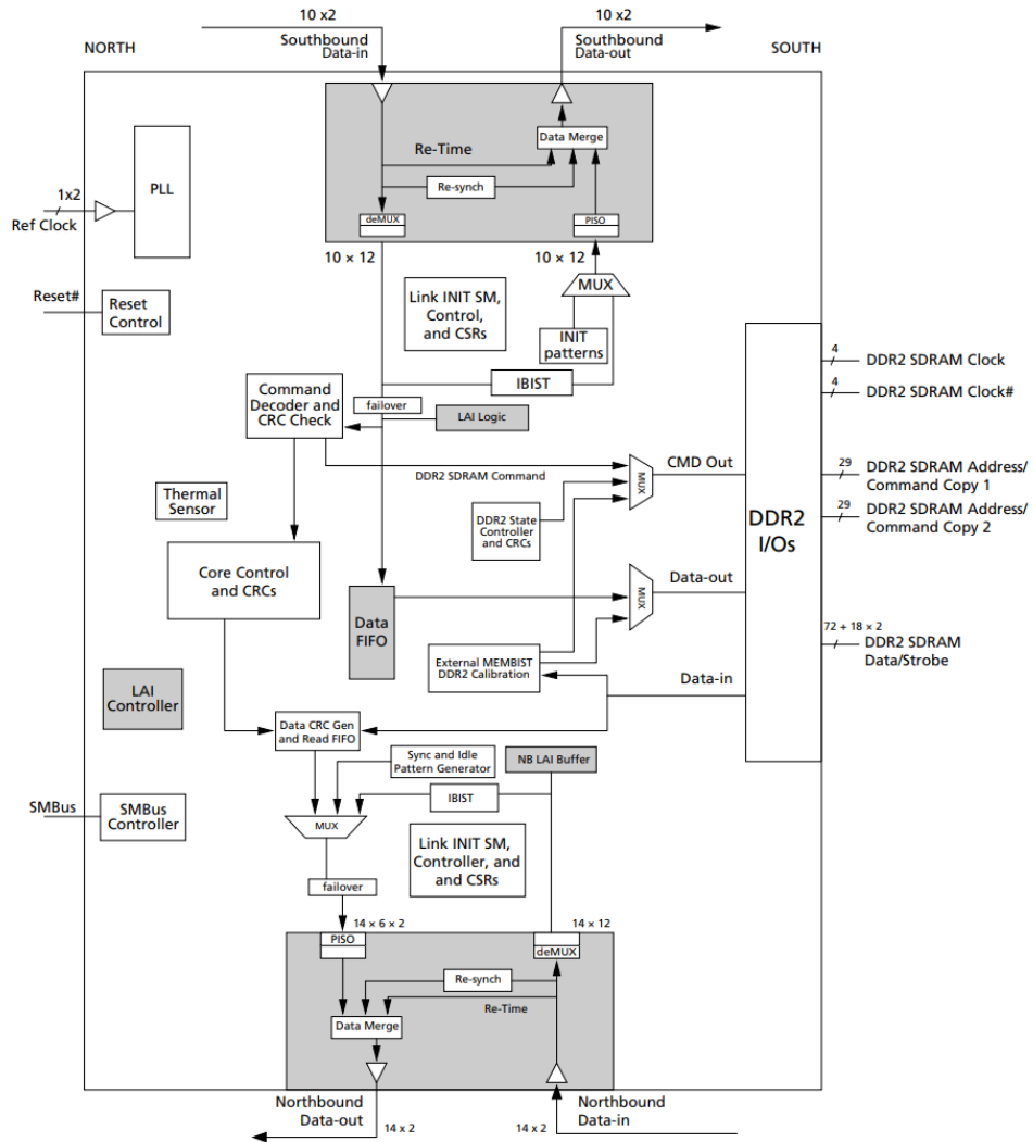
Figure 4: AMB Functional Block Diagram
