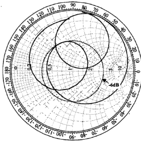
b) Smith Chart.
